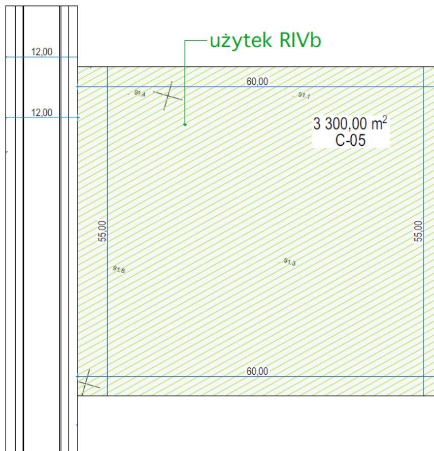
PARAMETRY DZIAŁKI
